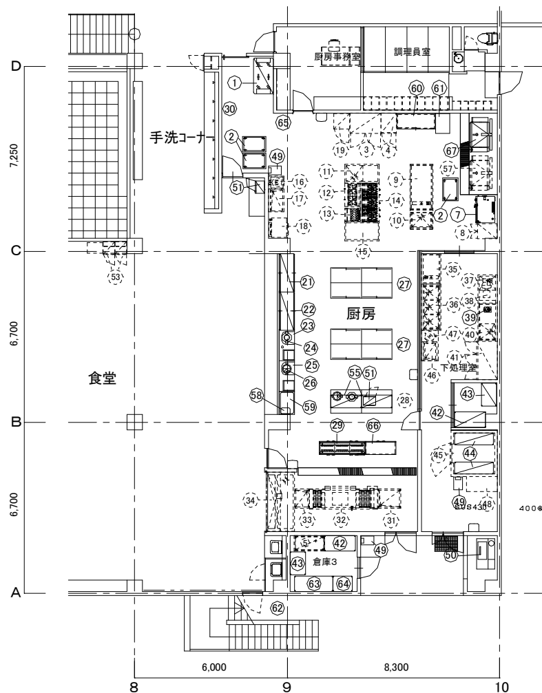
調理場配置図（救護施設丸山荘1号館1階）
